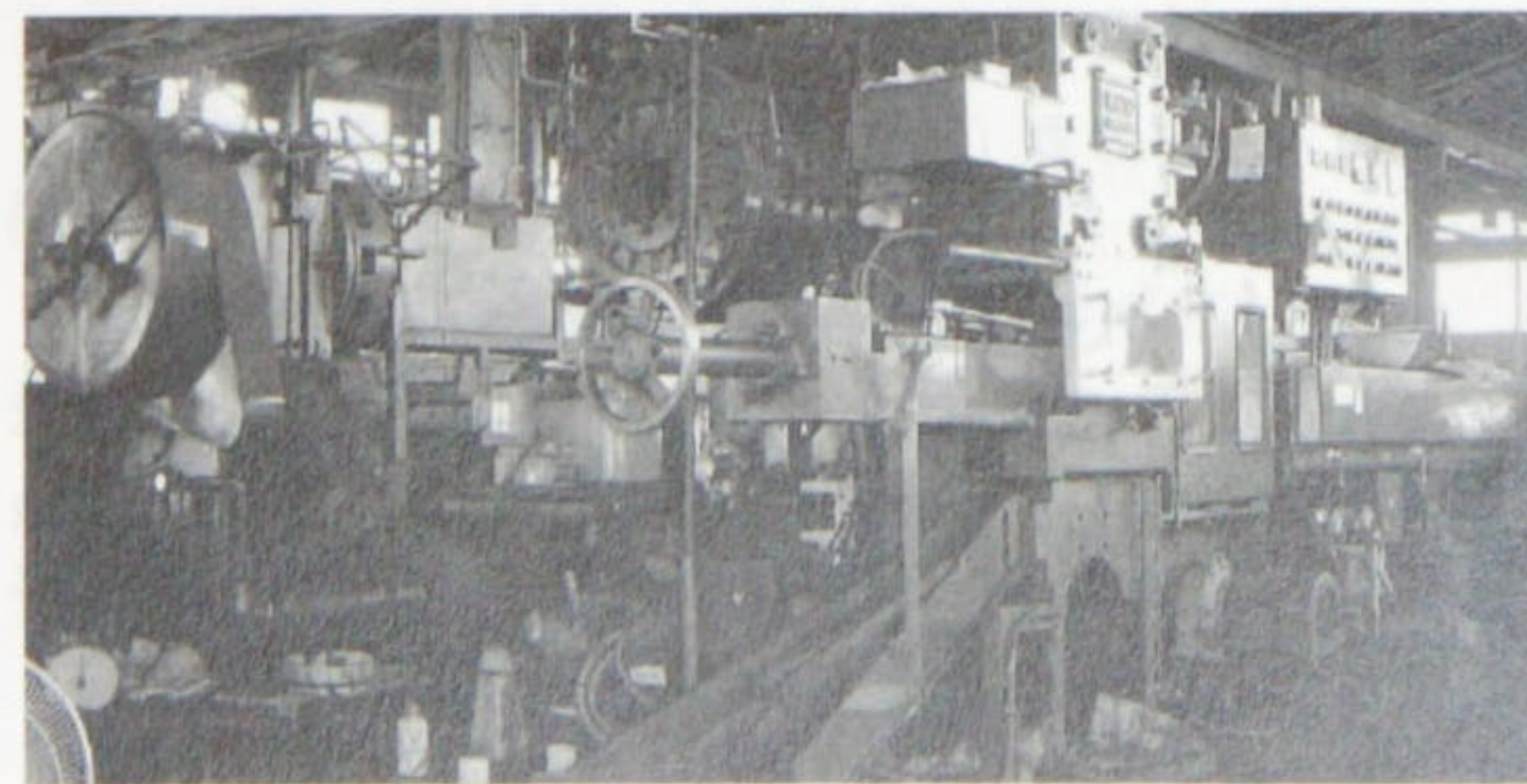
100T全自動丸棒切断機
